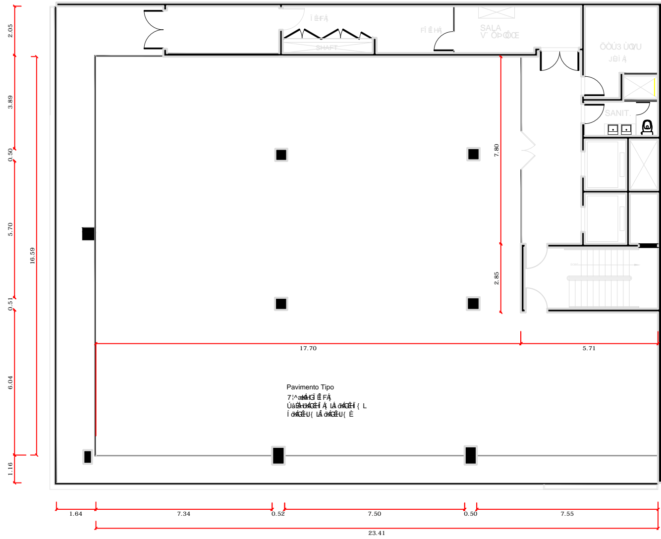
PLANTA BAIXA - PAV. TIPO
